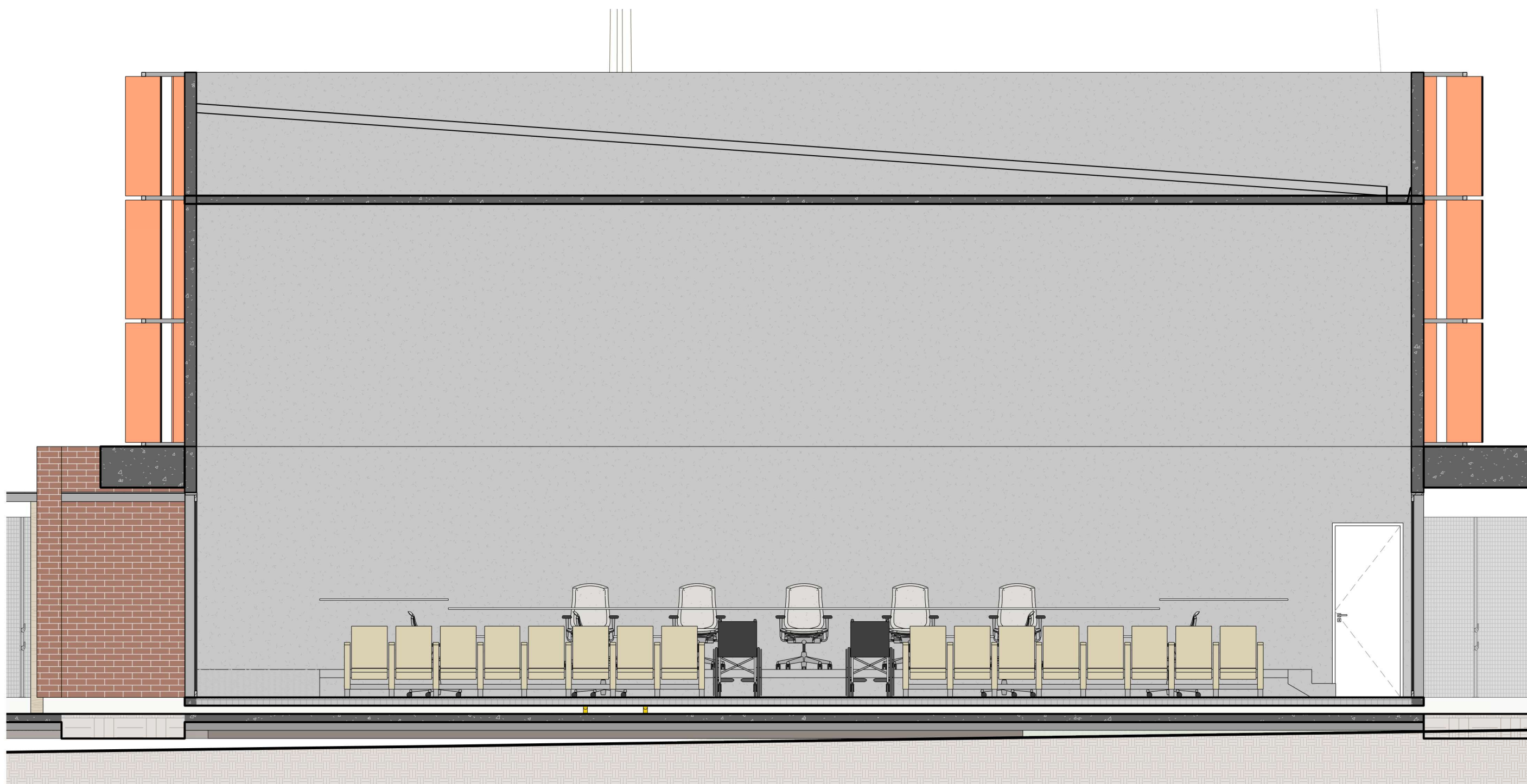
2 Corte DD ESCALA: 1:50
