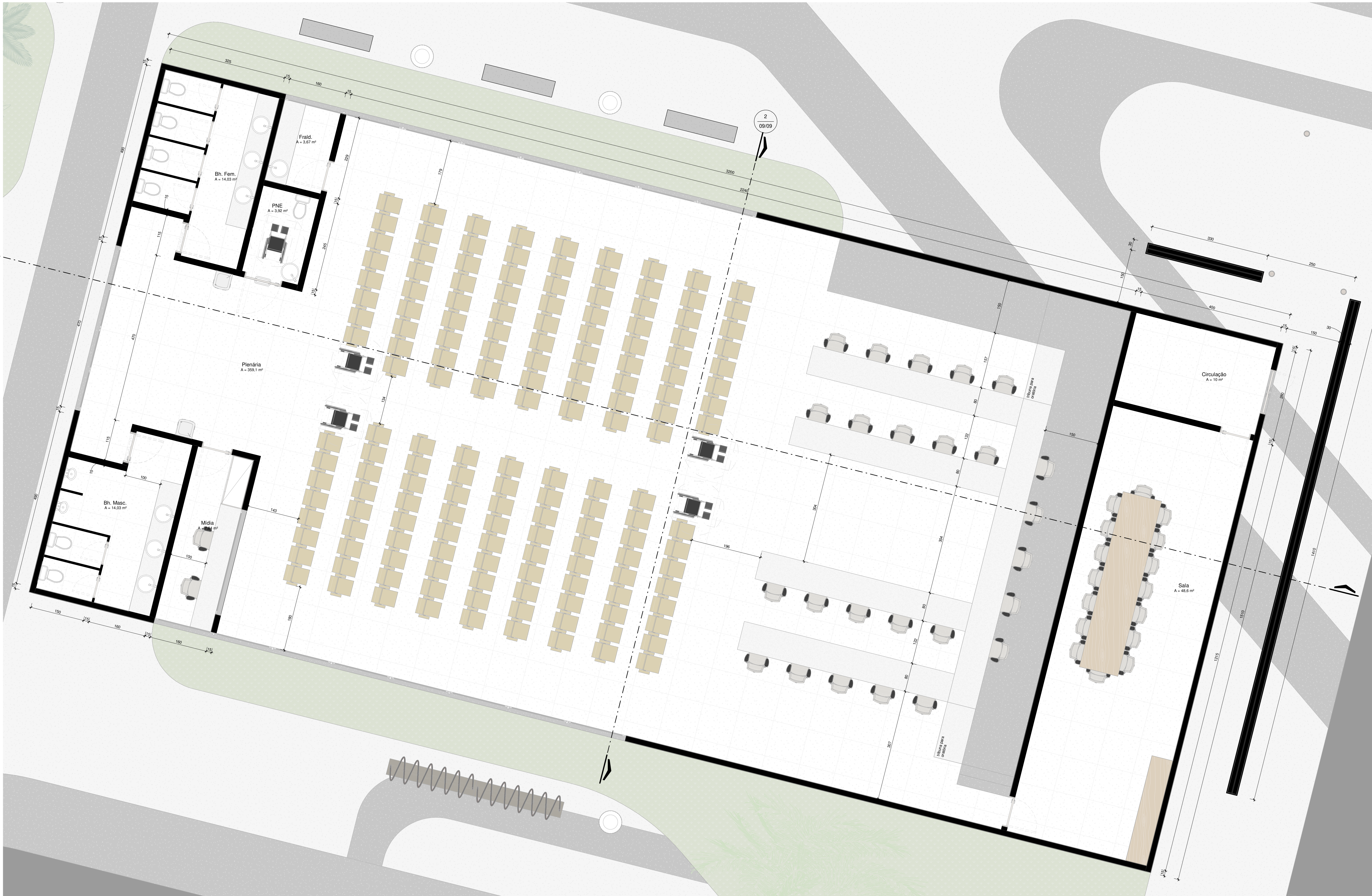
1 Térreo - Plenária ESCALA: 1:50
