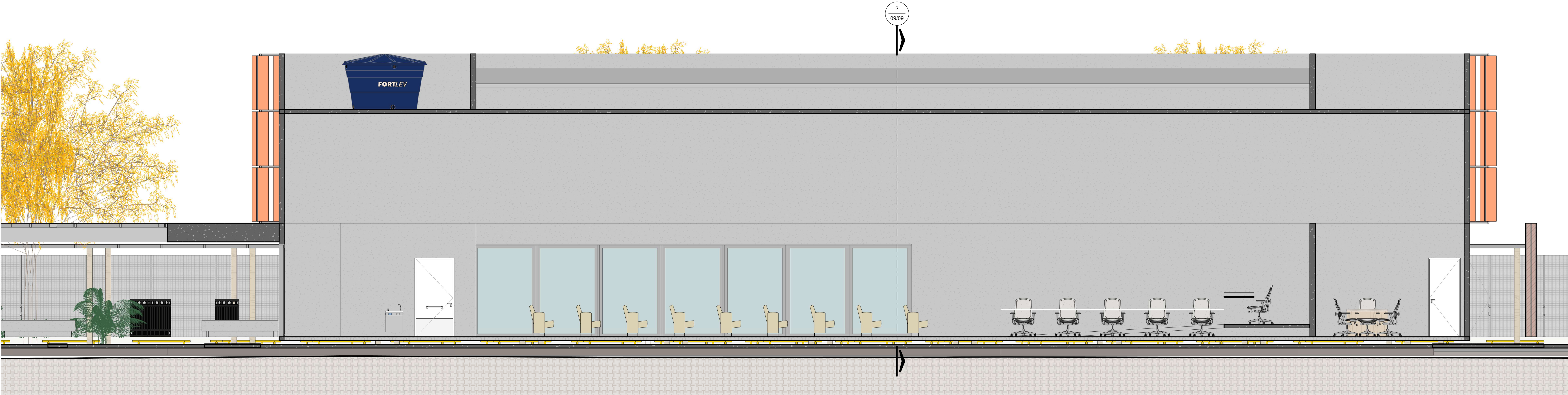
2 Corte CC ESCALA: 1:50
