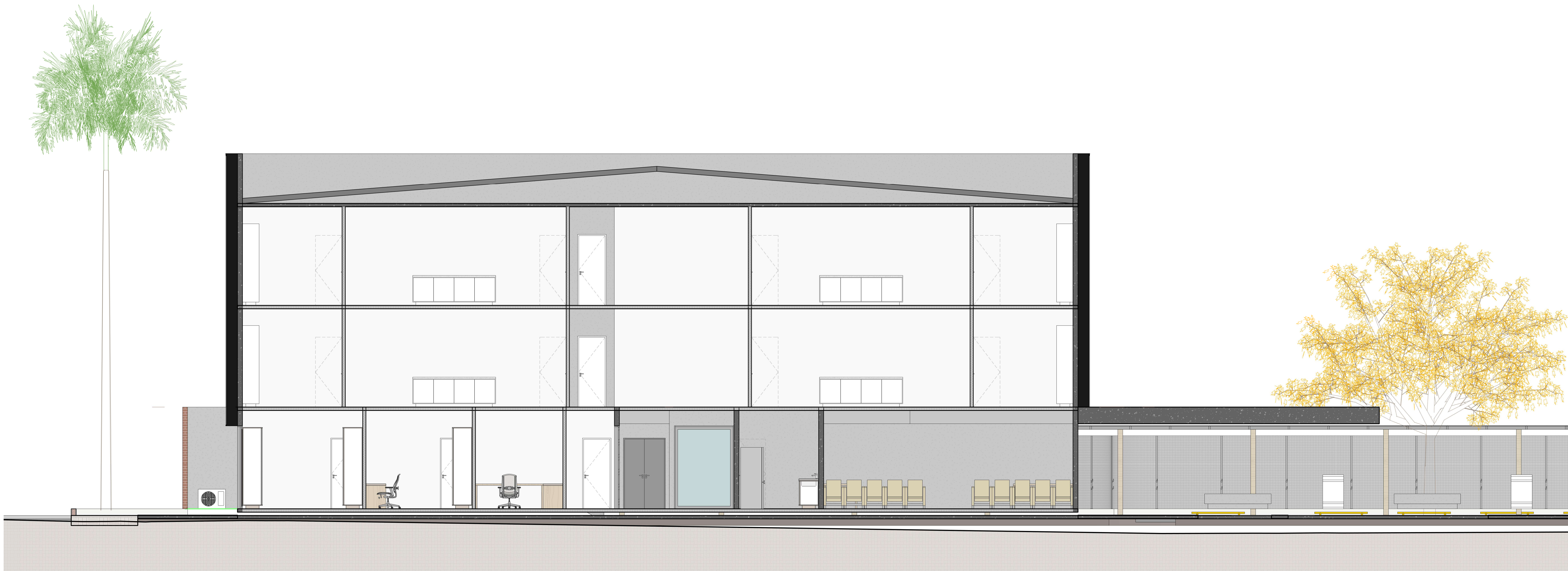
1 Corte AA ESCALA: 1:50
